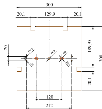
Détails plateforme supérieure épaisseur : 50mm
