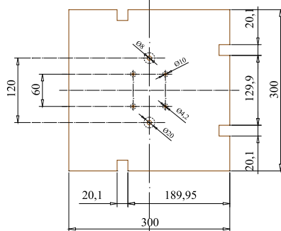
Détails plateforme inférieure épaisseur : 50mm
