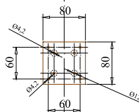
Détails embase épaisseur : 22mm
