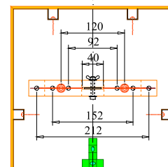
Détails chevron - potence
